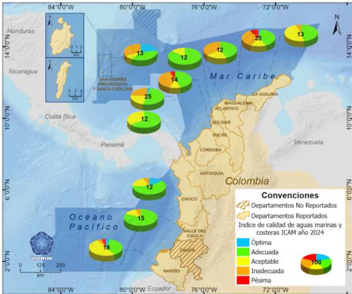
Figura 4. Representación del índice de calidad de s marinas y costeras – ICAM evaluado en los departamentos costeros de los litorales Caribe y Pacífico colombianos en el año 2024. El número en la gráfica indica el total de registros reportados. Elaborado por Janneth Andrea Beltrán. Labsis-INVEMAR.
